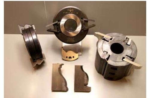
Diverse profielen
